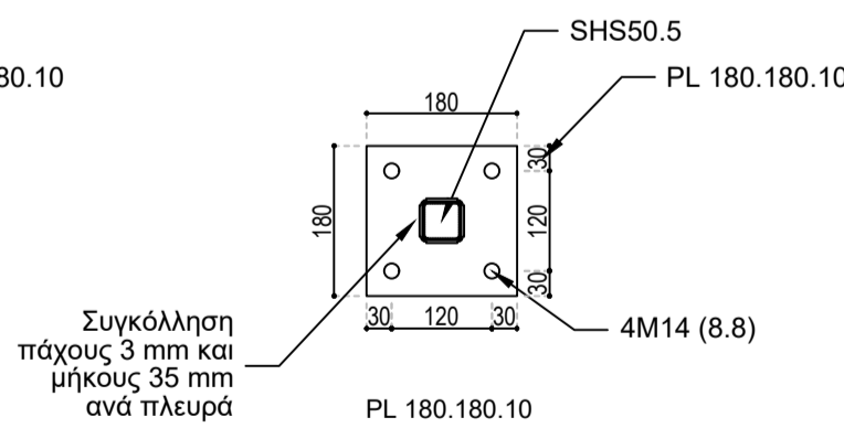
ΤΟΜΗ 2-2 ΚΛΙΜΑΚΑ 1:10
