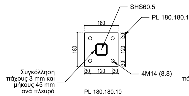
ΤΟΜΗ 1-1 ΚΛΙΜΑΚΑ 1:10
